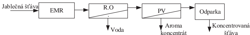
Obr. 3.4 Membránový proces spojený s PV k získání přírodního aroma a koncentráту jablečného džusu
