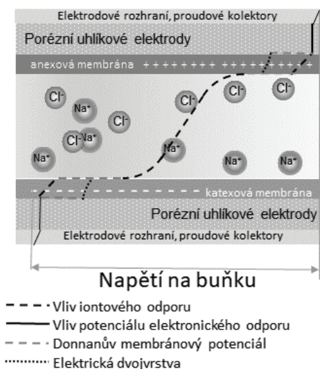
Obr. 5.5 MCDI napěťový profil komory
