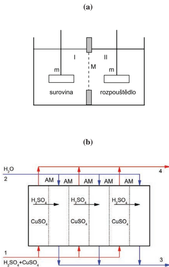
Obr. 4.3 Schéma (a) vsádkové a (b) kontinuální difuzní dialýzy; I, II – části cely, M – membrána, m – míchadlo; 1 – nástřík, 2 – rozpouštědlo, 3 – dialyzát, 4 – difuzát
