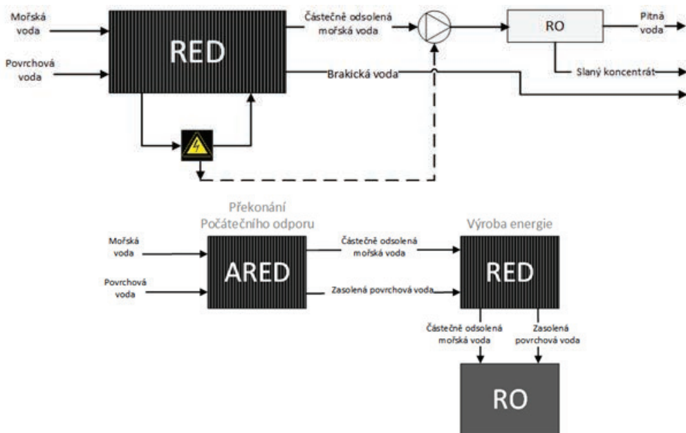
Obr. 5.8 Schéma hybridního procesu včetně ARED a RED jako kroků před odsolování pomocí RO. Znečištěná voda je zde preferovaným zdrojem málo slané vody, která slouží jako koncentrační roztok pro ionty z mořské vody [21]
