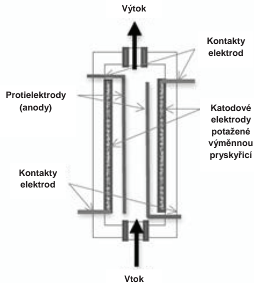
Obr. 5.4 Princip elektrochemické výměny iontů [5]
