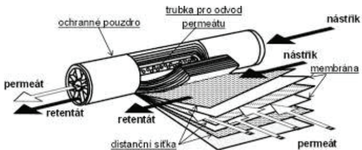
Obr. 1.9 Schéma spirálně vinutého membránového modulu [32]
