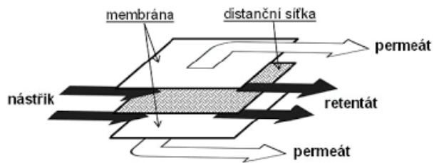
Obr. 1.7 Schéma deskového membránového modulu [30]
