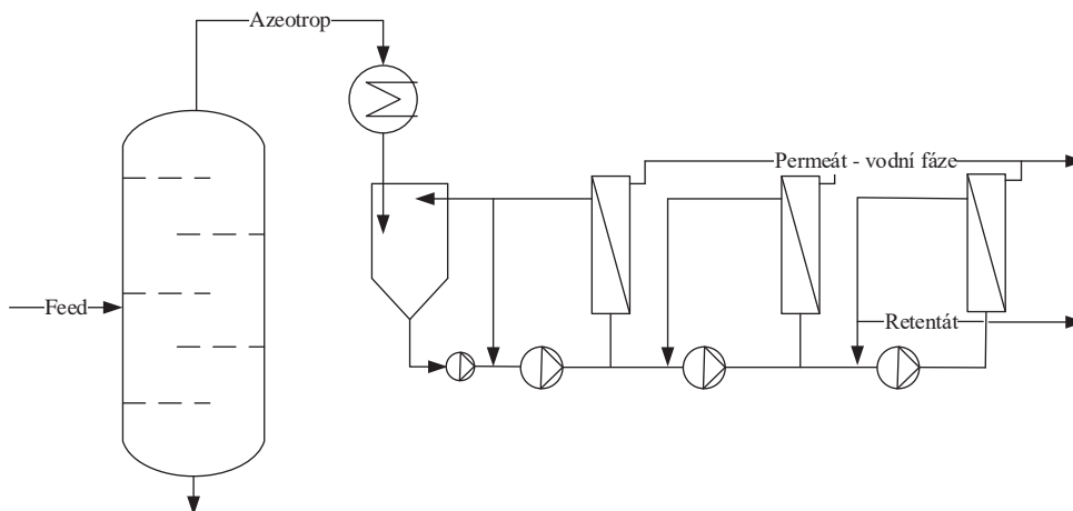
Obr. 3.2 Schéma hybridního kontinuálního procesu destilační kolona – pervaporace
