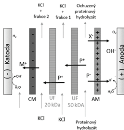
Obr. 5.7 EDUF pro získání antihypertenzních peptidů [11]
