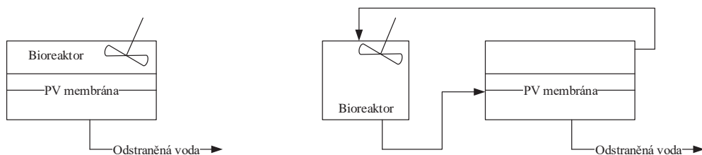
Obr. 3.6 Způsoby zapojení PV do enzymaticko-esterifikačního procesu
