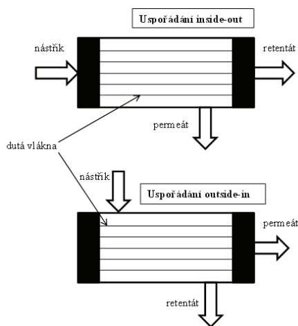
Obr. 1.13 Schéma uspořádání membránových modulů z dutých vláken
