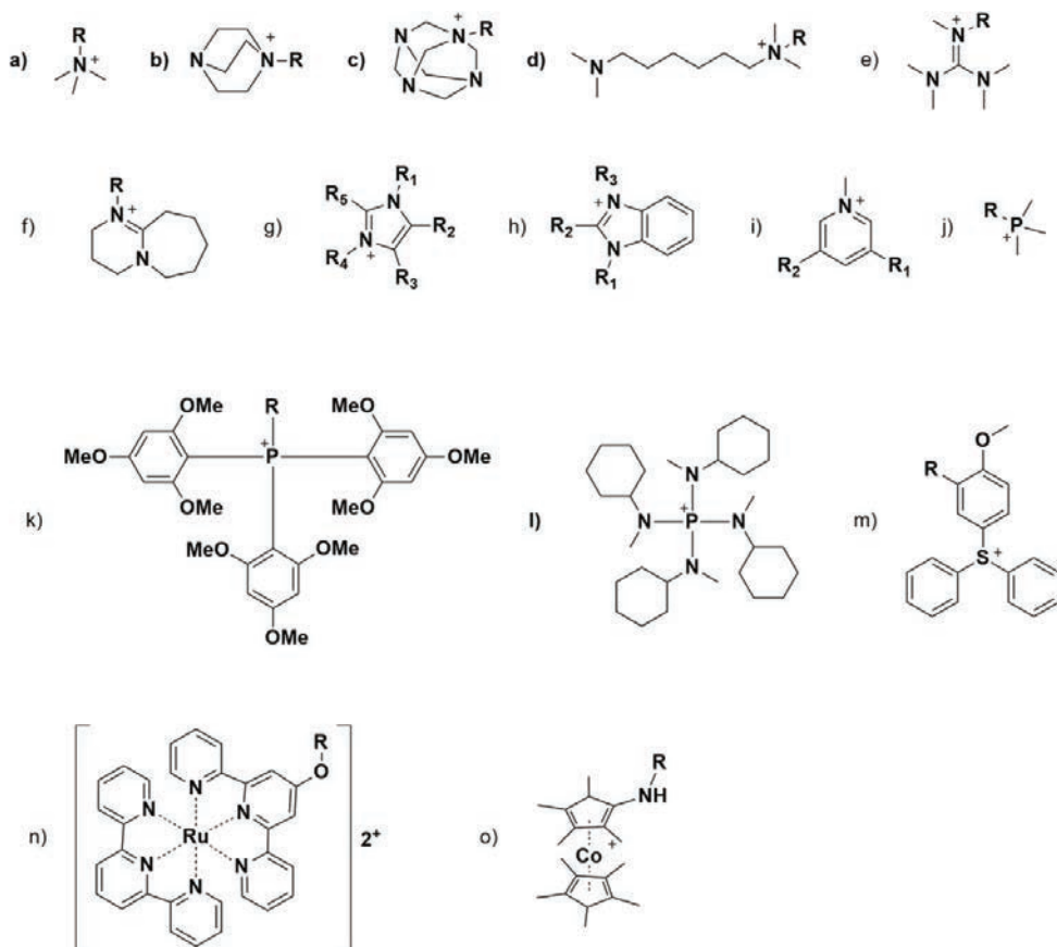
Obr. 1.5 Ukázka nejčastěji používaných anion výměnných funkčních skupin [10]
