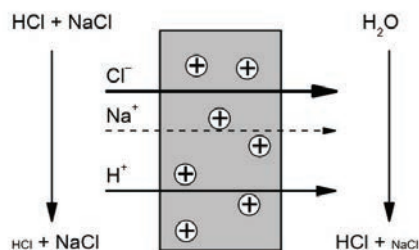
Obr. 4.1 Princip difuzní dialýzy s aniontově výměnnou membránou
