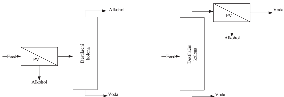
Obr. 3.3 Způsoby zapojení PV s destilační kolonou
