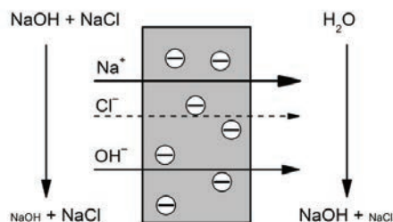
Obr. 4.2 Princip difuzní dialýzy s kationtově výměnnou membránou
