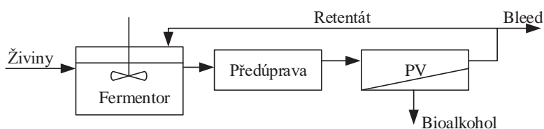
Obr. 3.5 Zapojení pervaporace do procesu fermentace
