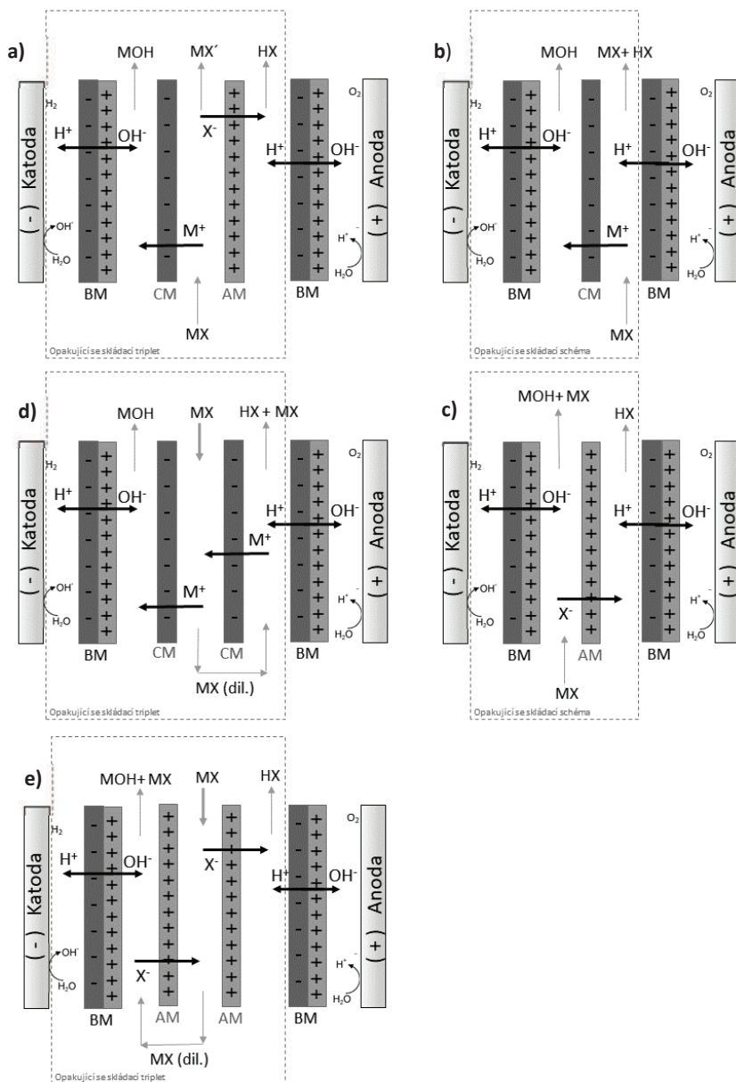
Obr. 5.3 Možnosti uspořádání EDBM
