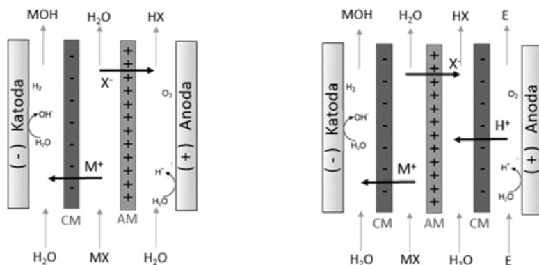
Obr. 5.2 Schémata možného uspořádání elektro-elektrodialýzy
