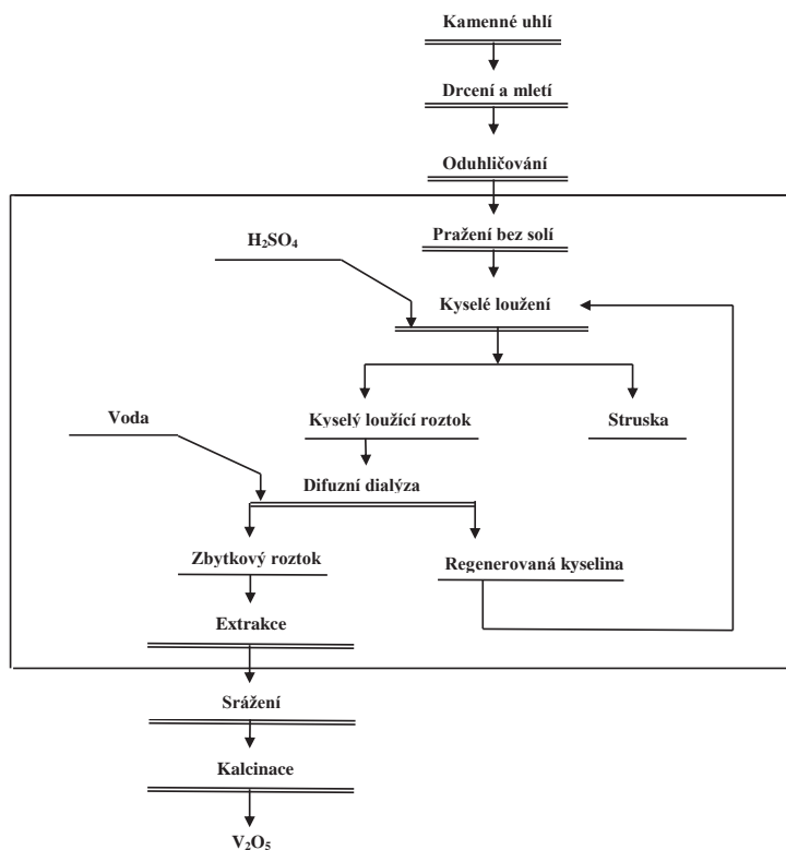
Obr. 4.4 Technologické schéma výroby vanadu z kamenného uhlí s aplikací DD [5]
