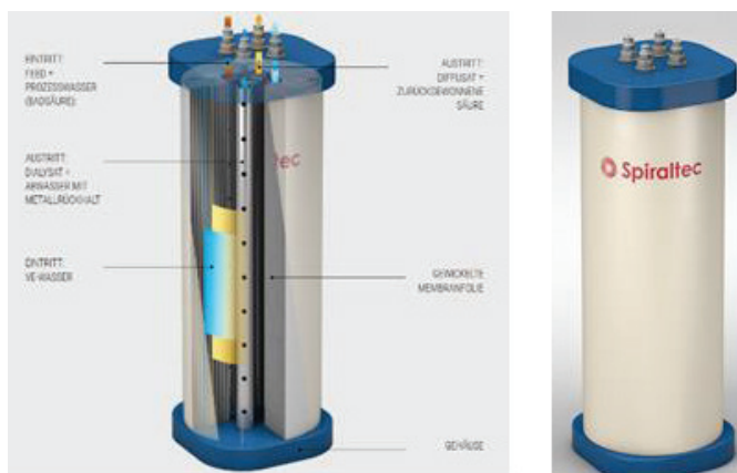
Obr. 4.9 Řez modulem firmy Spiraltec [35]
