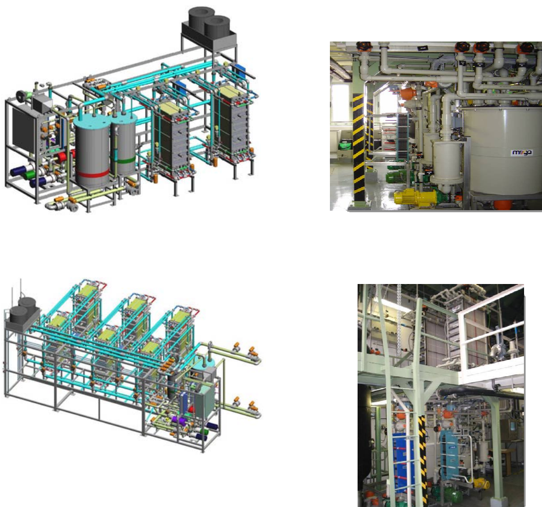
Obrázek 11: Fotografie membránové technologie firmy MEGA a.s. pro zpracování meziproduktů farmaceutického průmyslu v České republice
